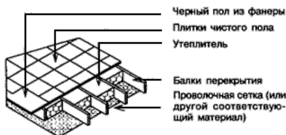
Перекрытие над неотапливаемым помещением, утепленное насыпным утеплителем
