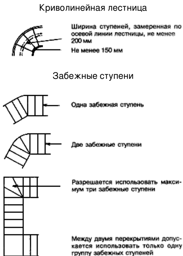
Рисунок 12-1 - Криволинейные лестницы и лестницы с забежными ступенями
