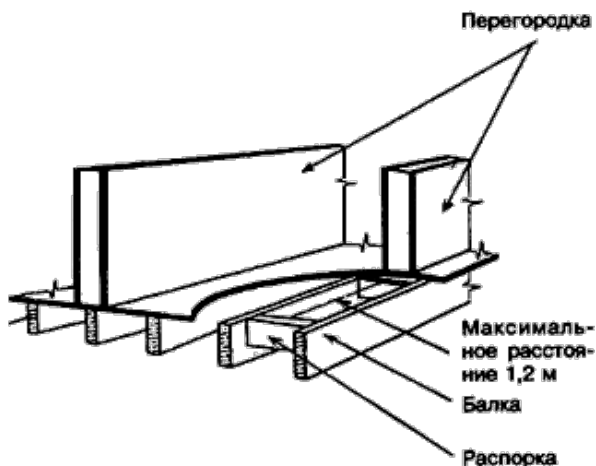
Рисунок 6-13 - Опираение перегородок
