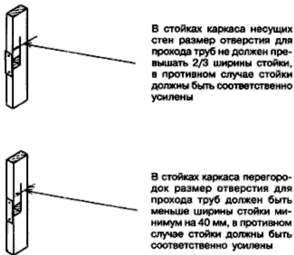
Рисунок 13-7 - Вырезы в стойках каркаса для прохода труб
