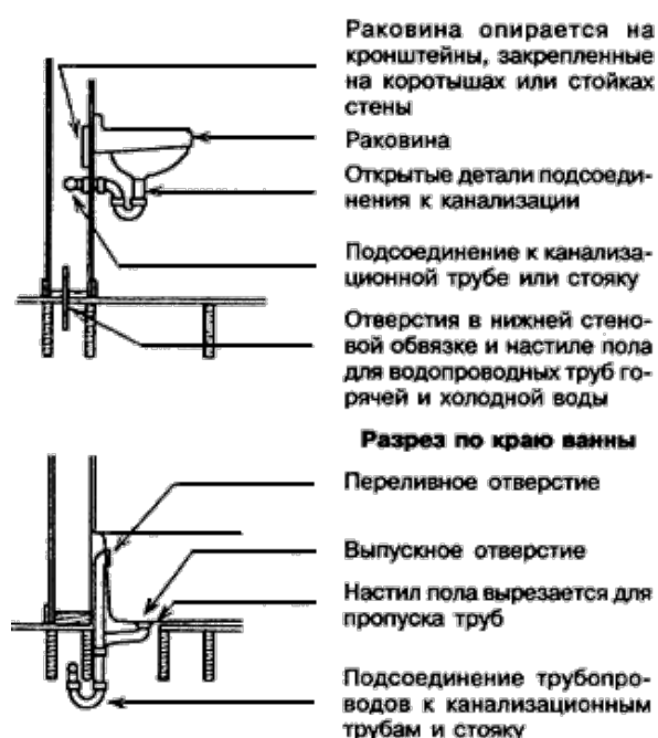
Рисунок 13-6 - Детали установки умывальника и ванны
