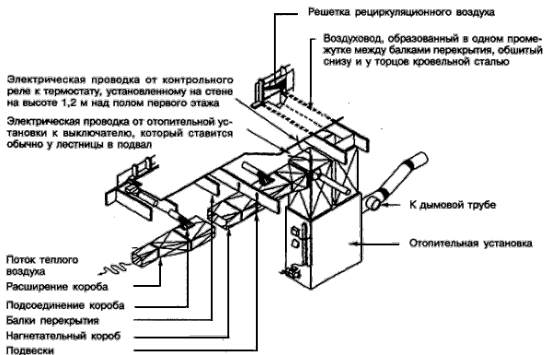
Рисунок 13-5 - Размещение отверстия для пропуска труб и электропроводки в балках перекрытия
