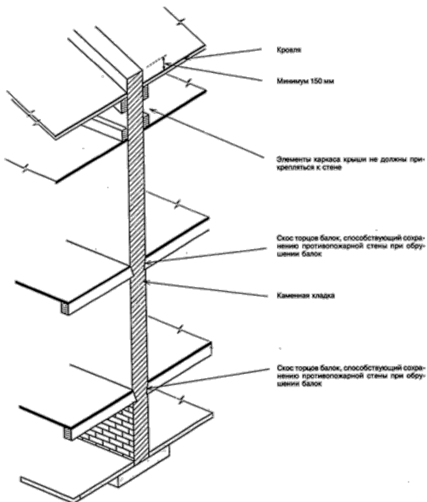
Рисунок 7-5 - Каменная противопожарная стена
