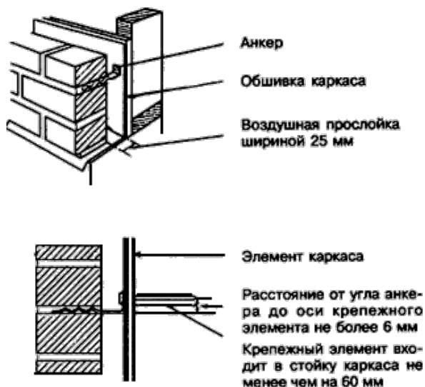
Рисунок 10-1 - Анкеры в каменной облицовке
